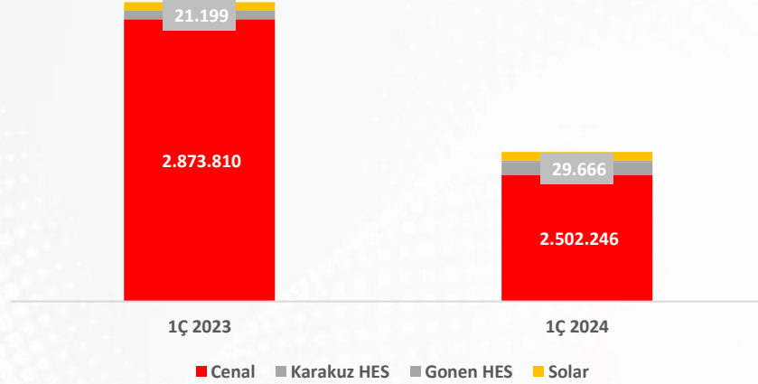
Net Elektrik Üretimi (KWh)*
